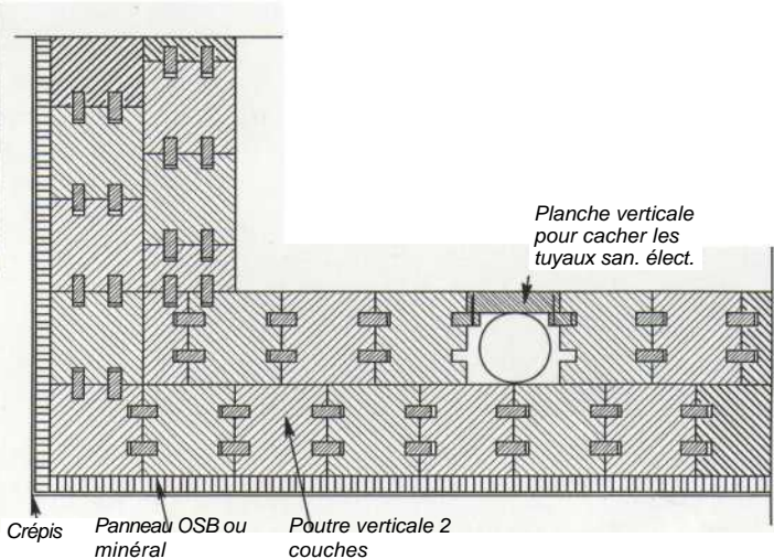
Détail d'un angle d'une maison en coupe horizontale. Aspect crépis. Dessinée le 3.3.04 par Pierre Messerli.
