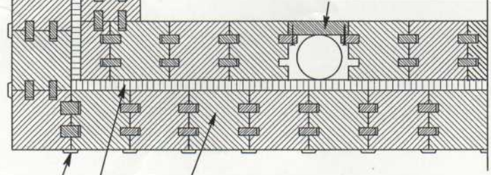
Détail d'un angle d'une maison en coupe horizontale Aspect bois. Dessinée le 3.3.04 par Pierre Messerli.
